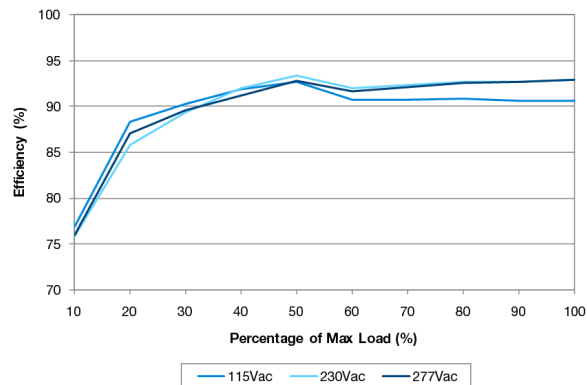
LNE-54V185W□
