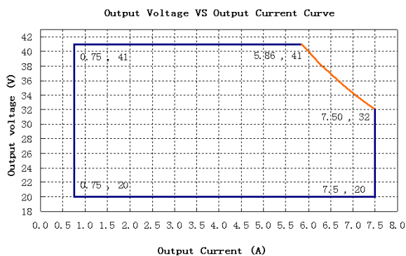
LDP-240X041
