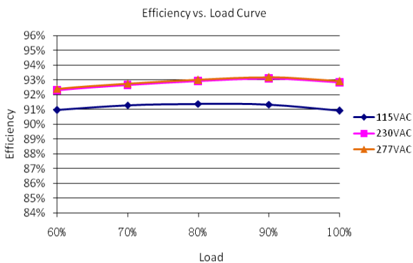
LDP-240X368-A (U=343V)
