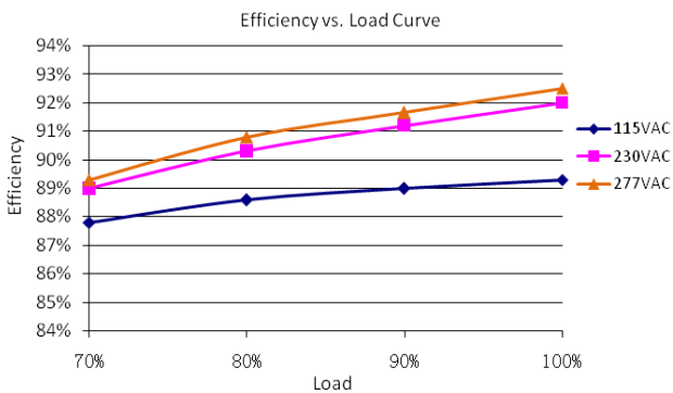
LDP-240X180-A (U=140V)
