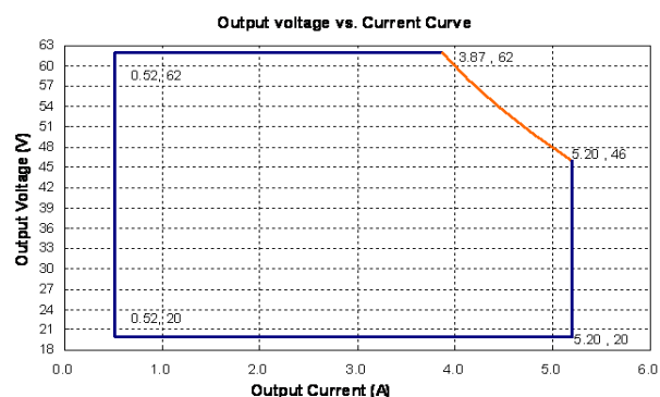
LDP-240X062
